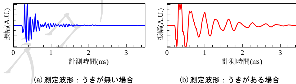
解説図2 各条件での測定波形
