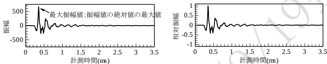
解説図 4 受信センサーの測定波形の例
